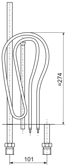
GREJAČ ZA BOJLER "TIKI" 10L ZA NISKU MONTAŽU
