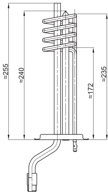
GREJAČ ZA BOJLER "MAGNOHROM" 5L ZA NISKU MONTAŽU
