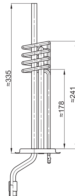
GREJAČ ZA BOJLER "MAGNOHROM" 10L ZA NISKU MONTAŽU
