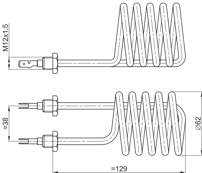
GREJAČ ZA BOJLER "TERMORAD" 10L ZA VISOKU MONTAŽU
