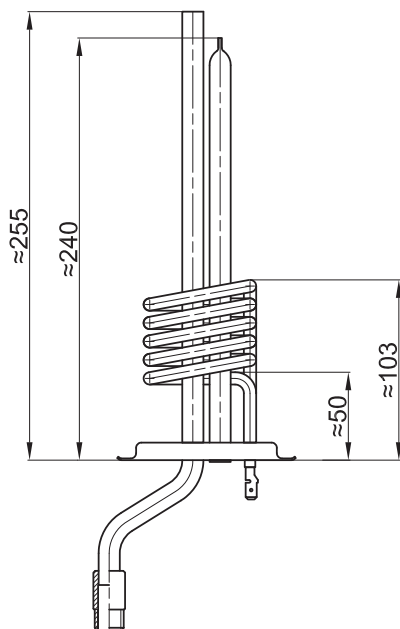
GREJAČ ZA BOJLER "MAGNOHROM" 5L ZA VISOKU MONTAŽU
