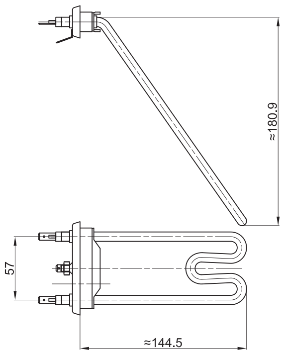
GREJAČ ZA VEŠ MAŠINU "BOSCH" SA RUPOM
