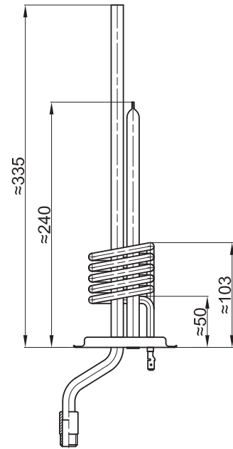
GREJAČ ZA BOJLER "MAGNOHROM" 10L ZA VISOKU MONTAŽU
