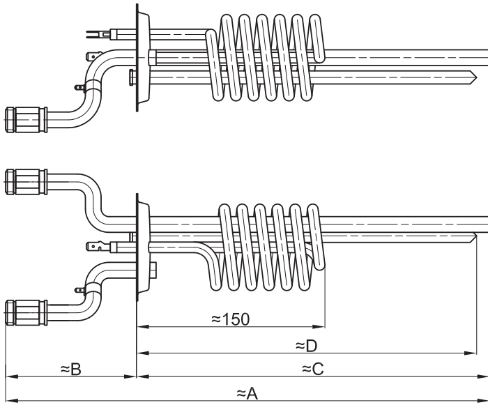
GREJAČ ZA BOJLER "KONČAR" NOVI TIP 5-10L ZA VISOKU MONTAŽU
